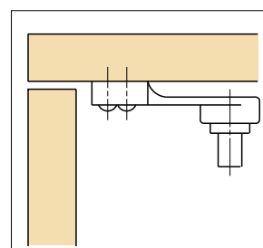
平座ブラケット
