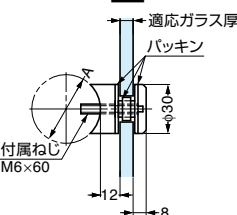
ガラス加工図
