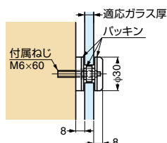
ガラス加工図
