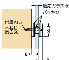
ガラス加工図
