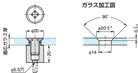
ガラス加工図
