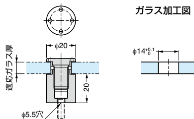
ガラス加工図
