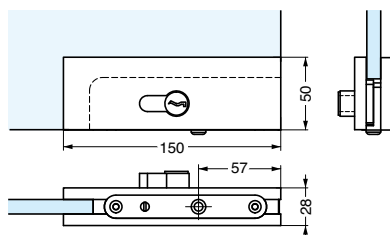
■ガラス加工図
