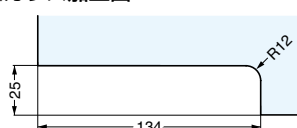
■ガラス加工図
