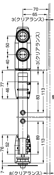
回 欄間ガラス取付仕様図
