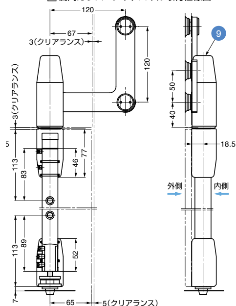
回 欄間ガラス+サイドパネル取付仕様図
