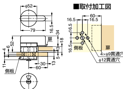
■取付加工図
