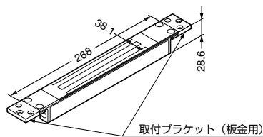
本体(枠取付)
