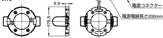
画像はばね取付タイプを示します。
