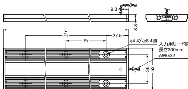
SL-T-100型、SL-T-24型(カバー脱着型) 取付ねじをカバーで隠すタイプ
