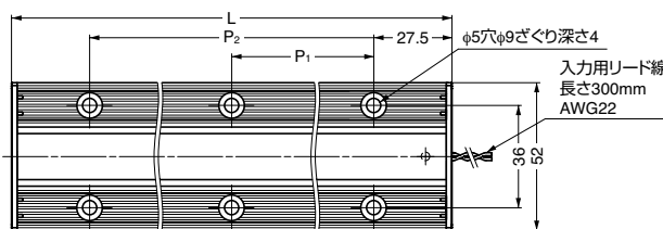
SL-T-24型(カバー一体型) カバーの上からねじで取り付けるタイプ
