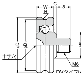
■ねじ軸仕様
