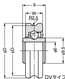
■内軸穴仕様
