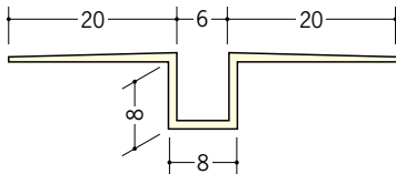
37119 ハット目地6 2.5m/ミルキー/40本入 3m/ミルキー/40本入
