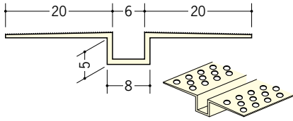
35223 ハット目地6×5穴あき 2.5m/ミルキー/50本入 3m/ミルキー/50本入
