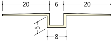
35221 ハット目地6×5 2.5m/ミルキー/50本入 3m/ミルキー/50本入
