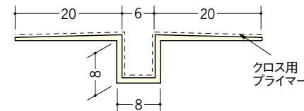
37172 ハット目地6クロス用プライマー付 2.5m/ミルキー/40本入 3m/ミルキー/40本入
