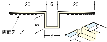
37141 ハット目地6テープ付 2.5m/ミルキー/40本入 3m/ミルキー/40本入
