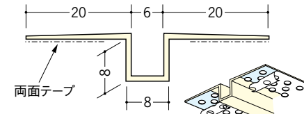
37145 ハット目地6穴あき+テープ付 2.5m/ミルキー/40本入 3m/ミルキー/40本入
