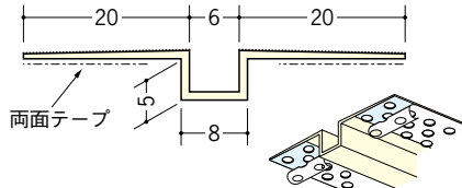
35224 ハット目地6×5穴あき+テープ付 2.5m/ミルキー/50本入 3m/ミルキー/50本入
