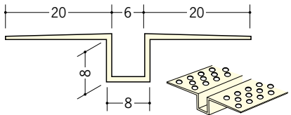
37142 ハット目地6穴あき 2.5m/ミルキー/40本入 3m/ミルキー/40本入
