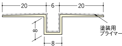
37144 ハット目地6塗装用プライマー付 2.5m/ミルキー/40本入 3m/ミルキー/40本入
