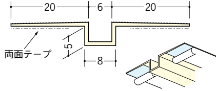
35222 ハット目地6×5テープ付 2.5m/ミルキー/50本入 3m/ミルキー/50本入
